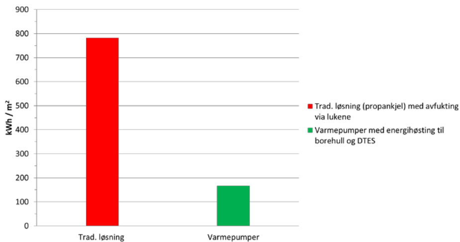
Figur 4. Energiforbruk over ett år for tradisjonell veksthusløsning på Mære (oppvarming med olje, gass, bio, etc.) og for varmepumpeanlegget med termisk energilagring i borehull.
