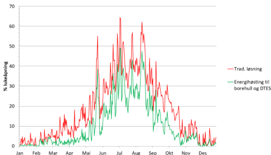
Figur 5. Gjennomsnittlig lukeåpning gitt i % over ett år for tradisjonell veksthusløsning (avfukking ved bruk av luker og økt varmpådrag) og ved bruk av varmepumper og avfukking med aerotempere.
