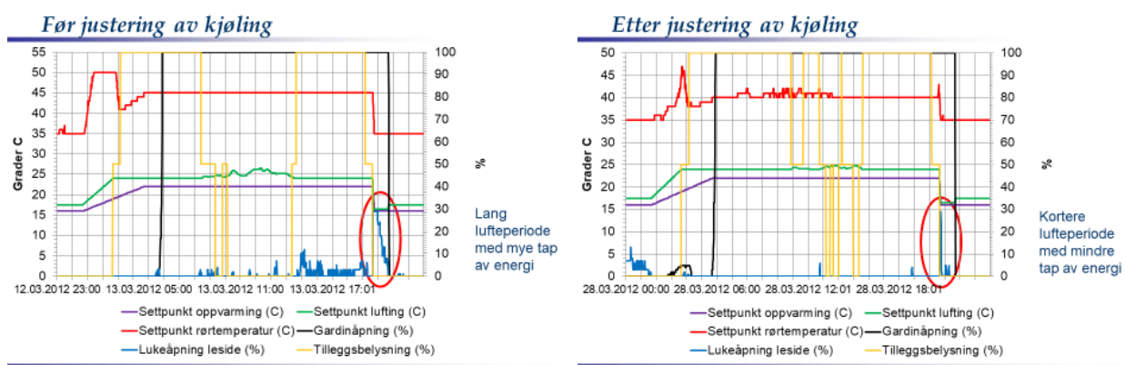
Figur 2. Grafer for settpunkt av oppvarming, rørtemperatur og lufting, i tillegg til åpning av lufteluker, gardinåpning og tilleggsbelysning før og etter justering av kjøling.
